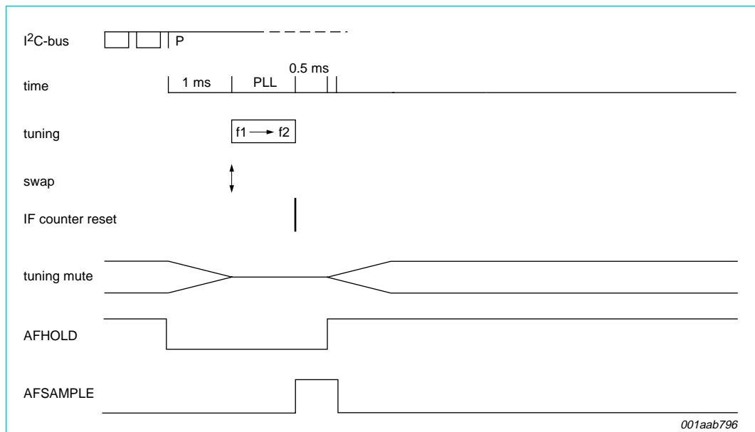
Fig 16. Jump mode
